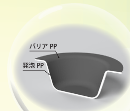
発泡PP/PBPラミ成形
