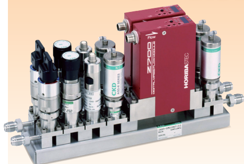
▲集積化ガス供給システム IAGDシリーズ
