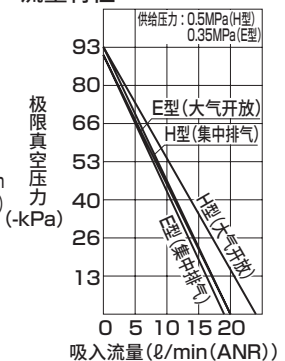
流量特性
