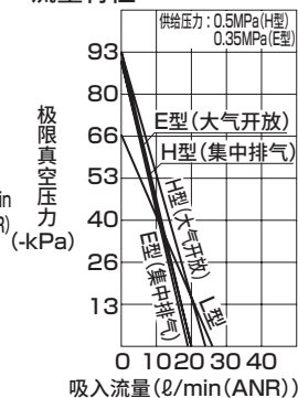
流量特性
