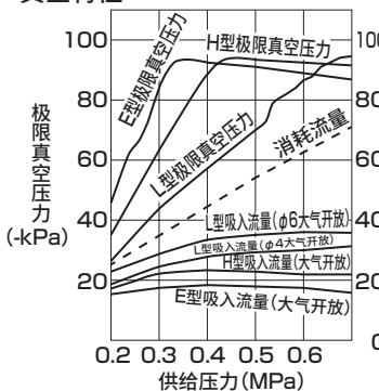
真空特性
