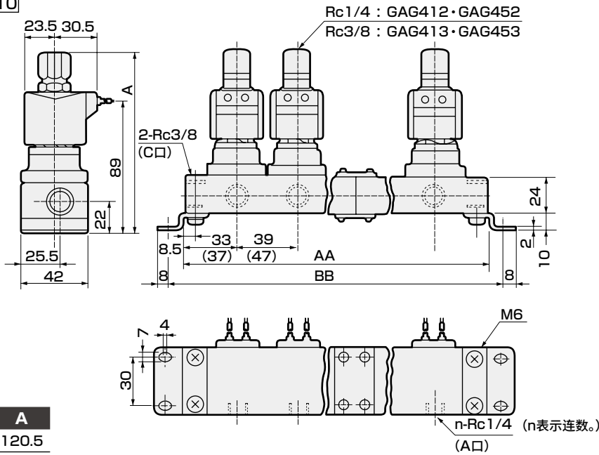
外形尺寸图：GAG41※・45※系列
