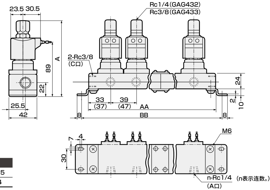
外形尺寸图：GAG432・GAG433系列
