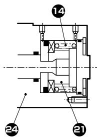
O(常开)型
