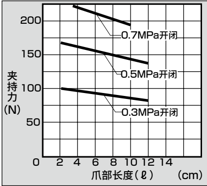
● HMF-G-25CS
