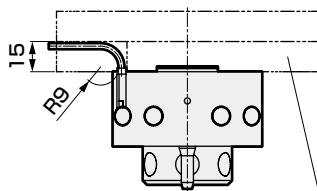
自动工具快换装置安装法兰(参考)
