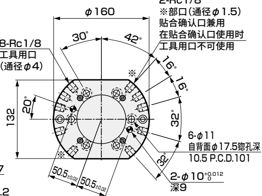
模块选择项1安装侧
