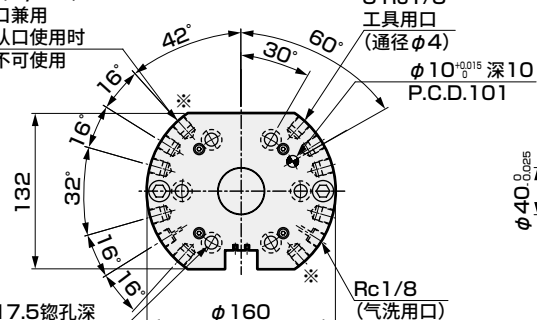
模块选择项1安装侧
