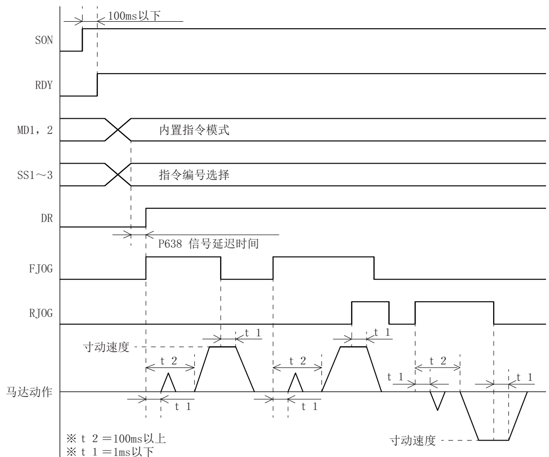
图5-5 寸动动作时序图
