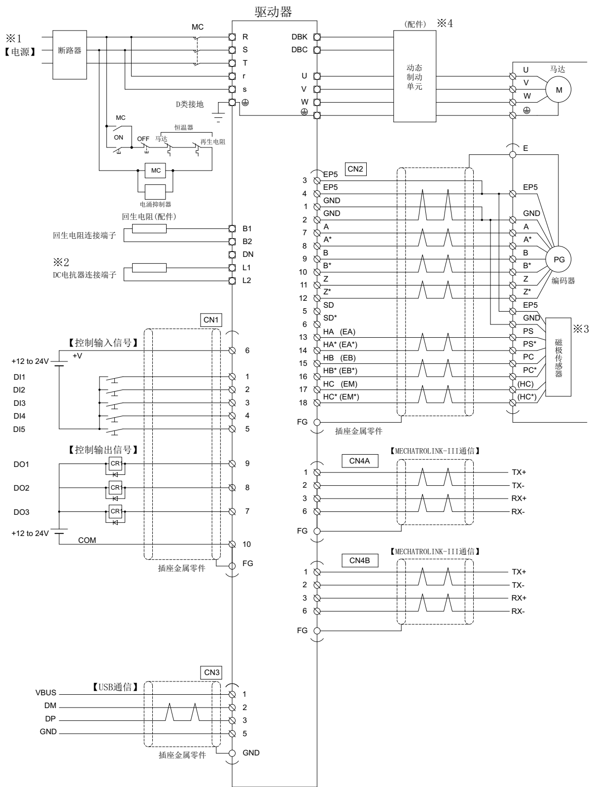
图3-1 外部连接图
