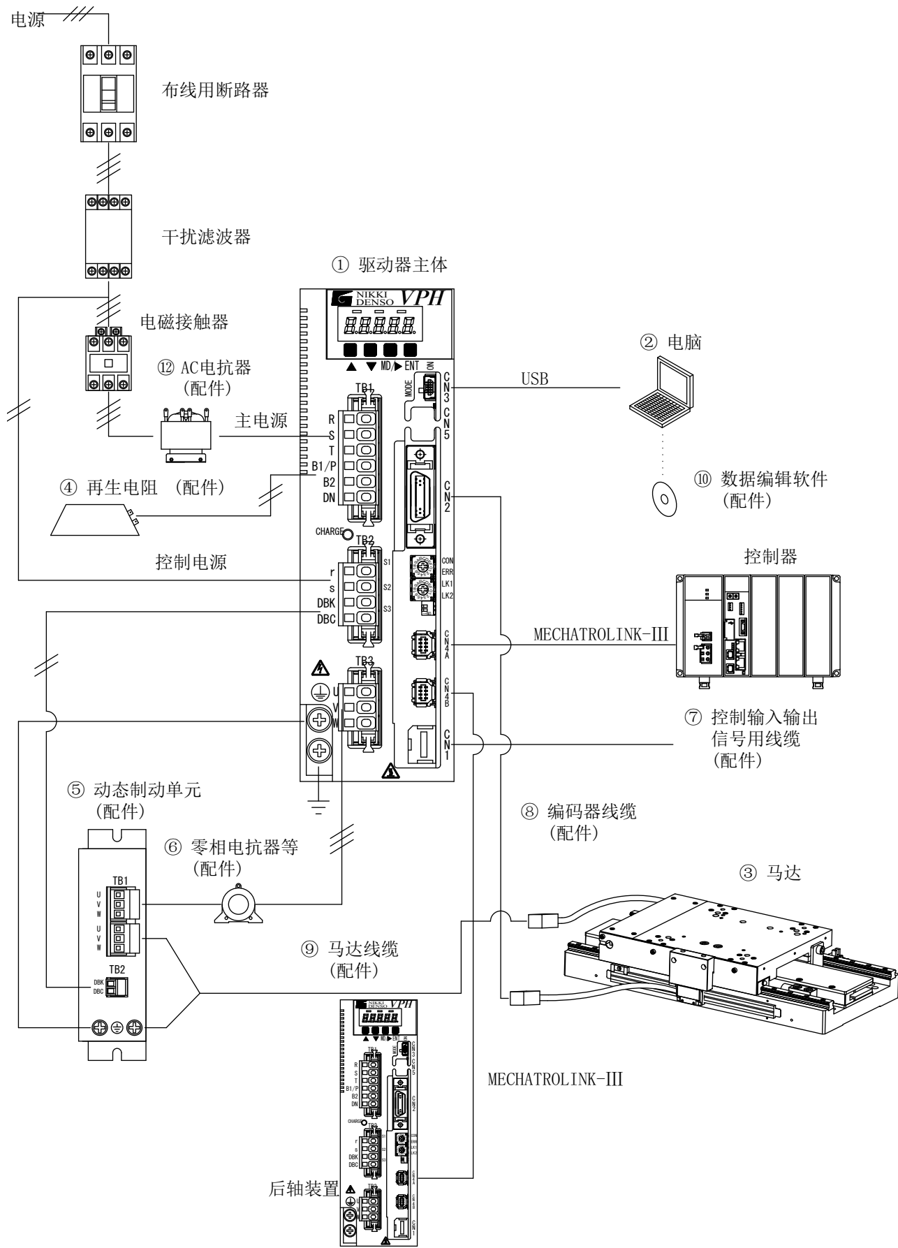
图1-1 800W级以下VPH HE类型 系统构成
