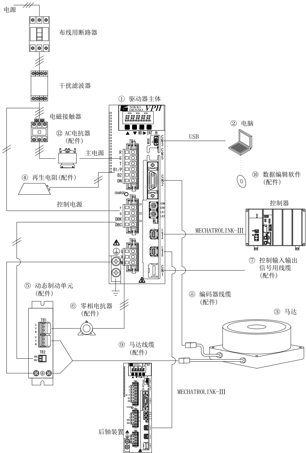
图1-1 800W级以下VPH HE类型 系统构成
