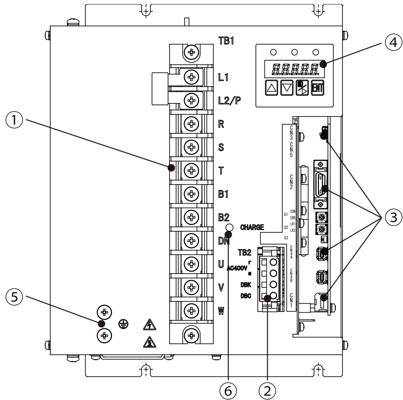
图13-14 400V 7kW驱动器主体正面图（Type7）
