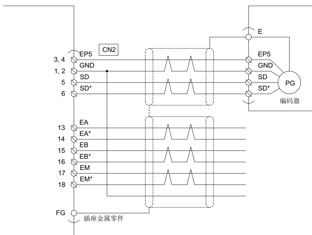
图3-2 串行编码器连接图
