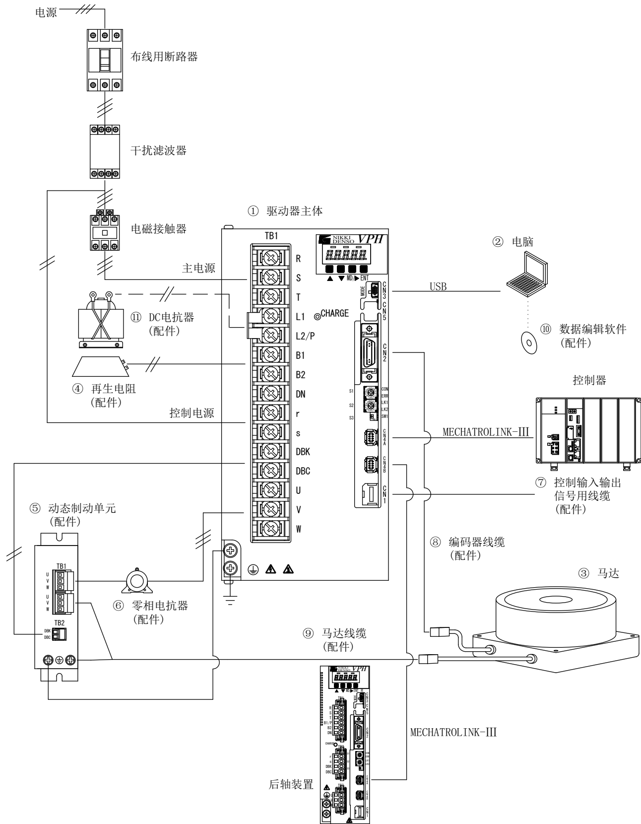
图1-2 1.5kW级以上VPH HE类型 系统构成
