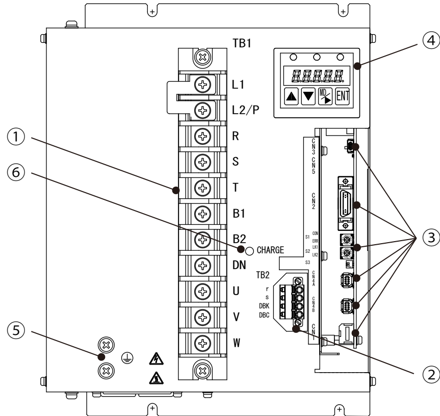
图13-10 200V 7kW驱动器主体正面图（Type5）
