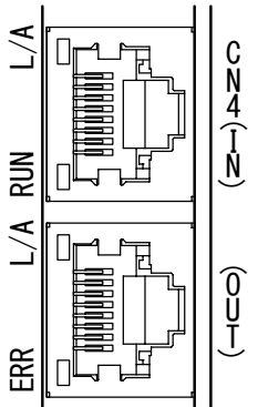
图1-4 状态LED
