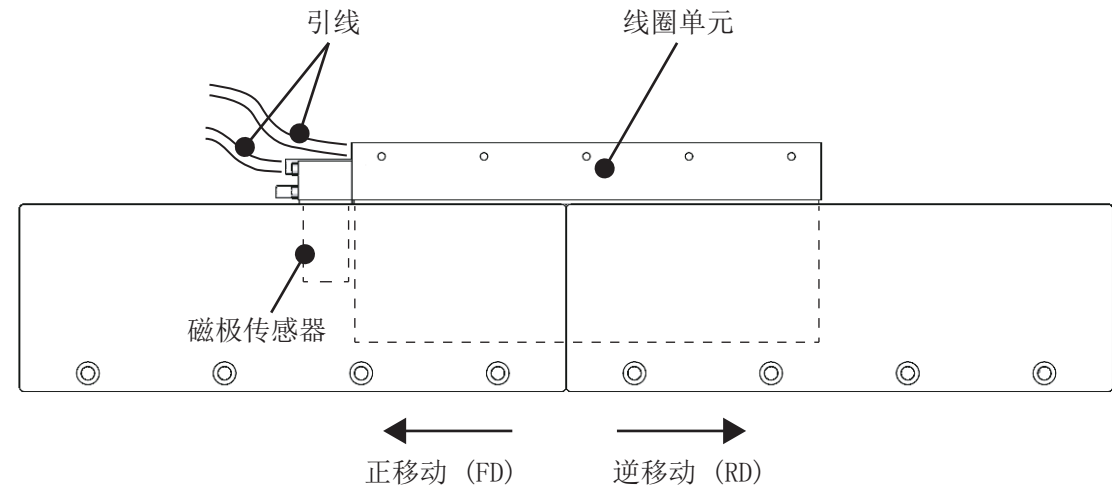
图4-1 线圈单元与磁极传感器的动作方向
