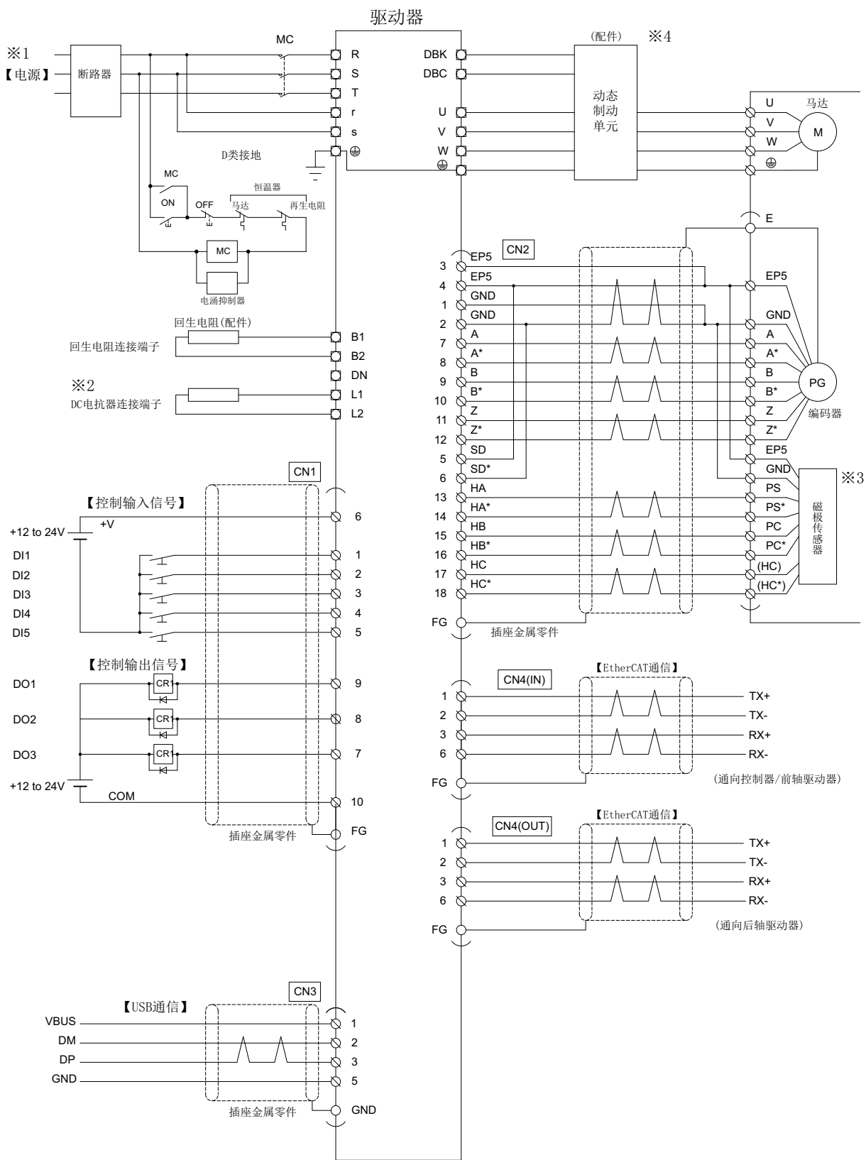
图3-1 外部连接图
