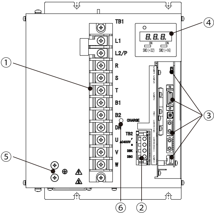
图12-14 400V 7kW驱动器主体正面图（Type7）
