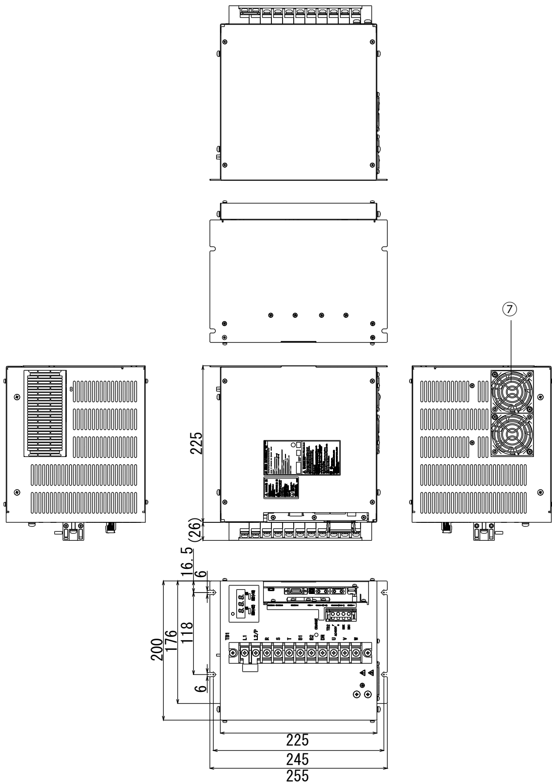
图12-13 400V 7kW驱动器主体外形图 (Type7)
