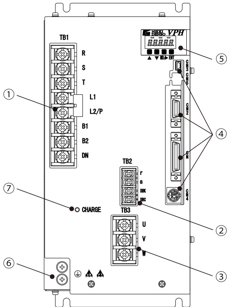
图13-8 3.3kW驱动器主体正面图（Type4）
