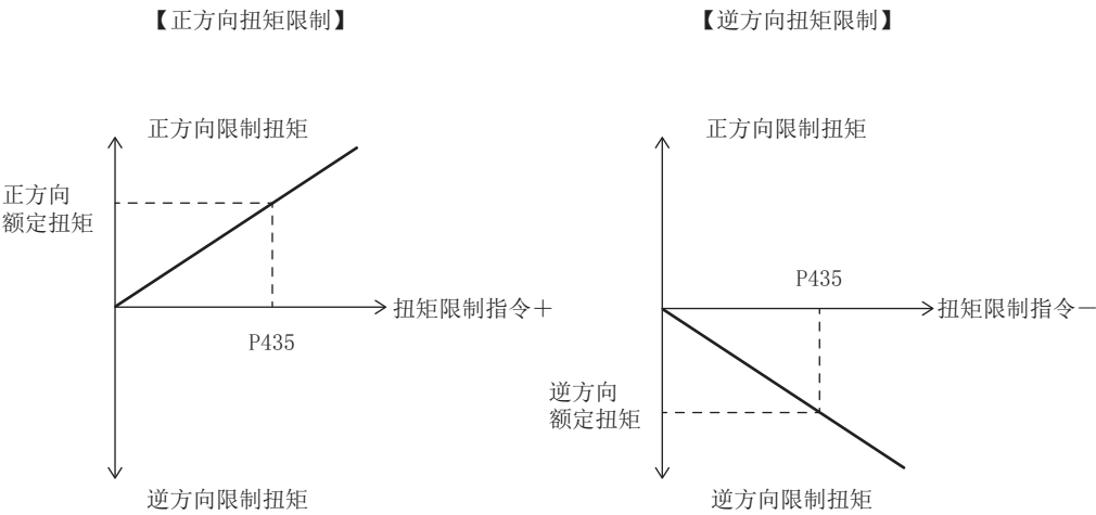
图5-13 基于模拟扭矩指令的扭矩限制
