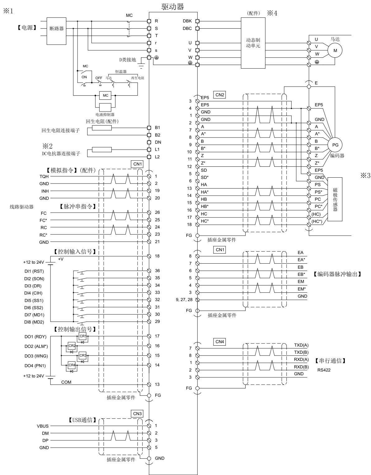
图3-1 外部连接图
