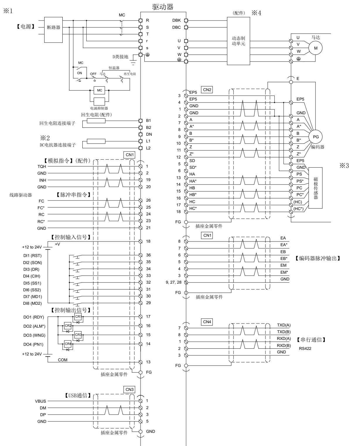
图3-1 外部连接图
