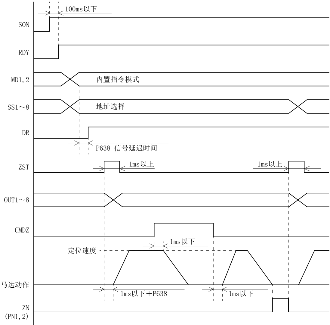
图5-31 INDX命令时序图
