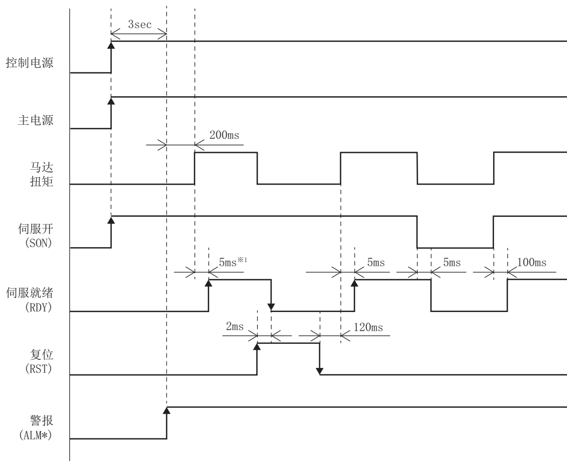
图2-11 时序图
