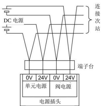
3. 分离单元电源和阀电源的连接
