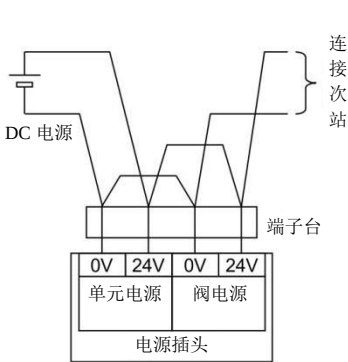
1. 单元电源和阀电源共用时
