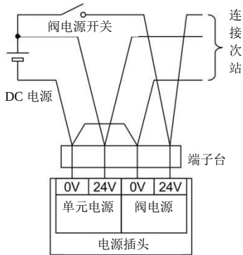
2. 切换阀电源 ON/OFF 的连接
