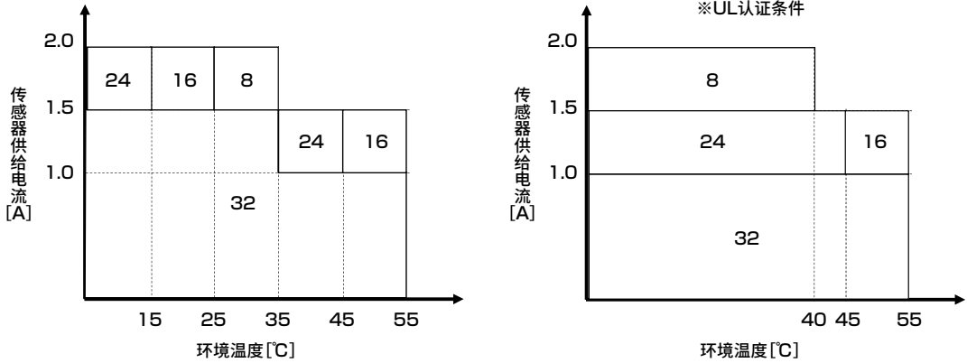
RT-XADGC32A/B的最大打开点数因环境温度和传感器供给电流而受到限制。请参阅以下图表。 (左：一般条件、右：UL认证条件)
