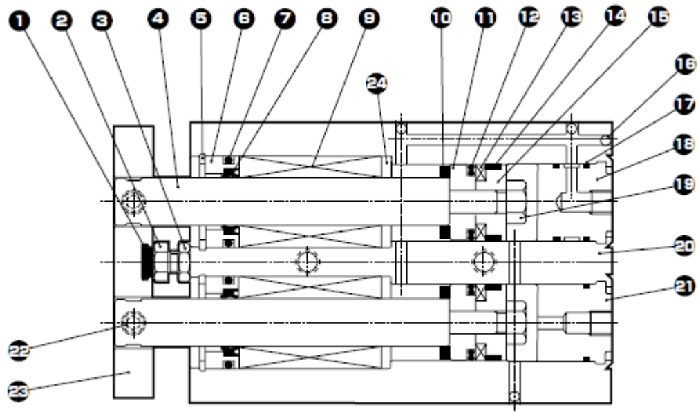
部件一览表
