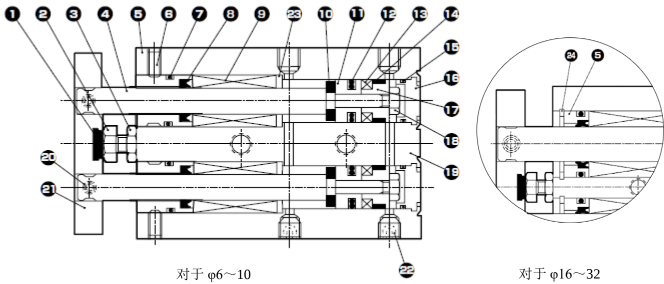
部件一览表
