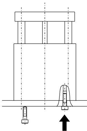
〈底面安装〉
