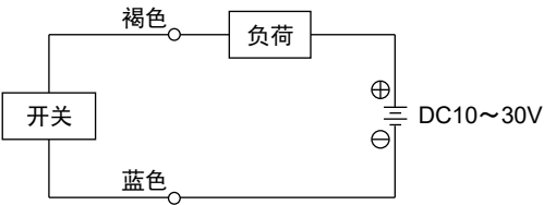
2 线式基本回路例
