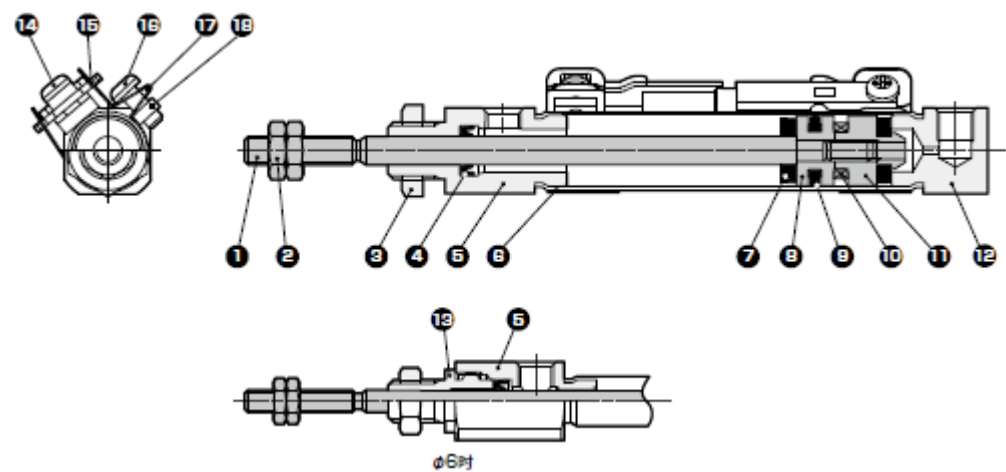
部件一览表
