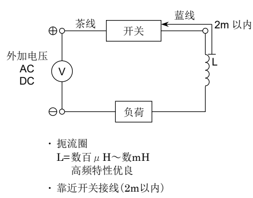
＜接线长度超过上表时的保护＞
