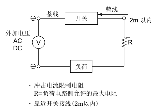
＜接线长度超过上表时的保护＞
