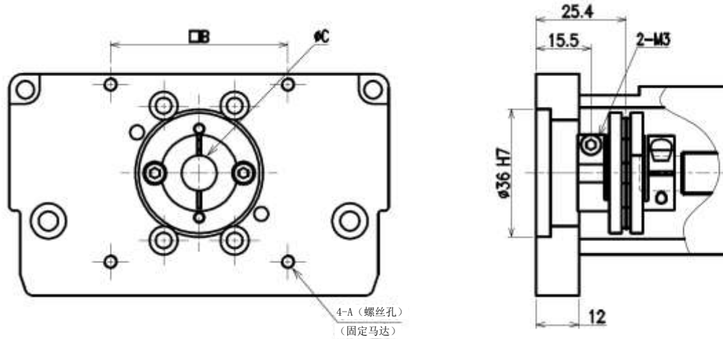
【ECS-12-※※※※※-E】 （马达大小：C <□60>）
