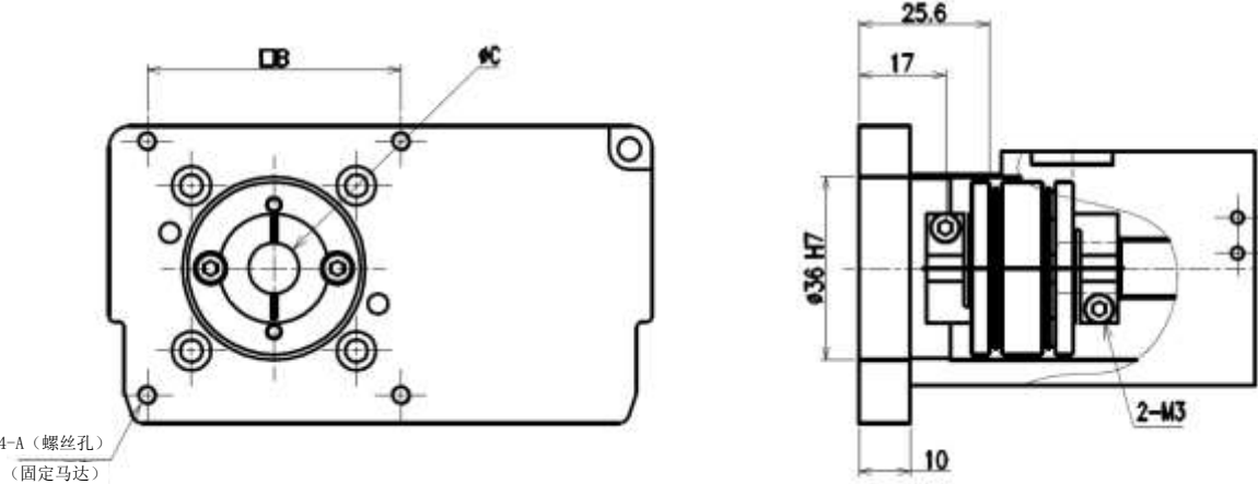
【ECS-10-※※※※※-E】（马达大小：C <□60>）
