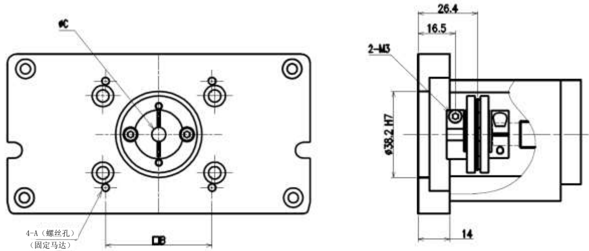
【ECS-14-※※※※※-E】（马达大小：B <□56>）
