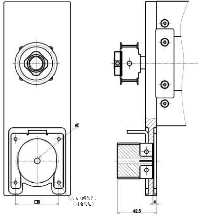
【ECS-14※※※※※- R/L/D】（马达大小：C <□60>）
