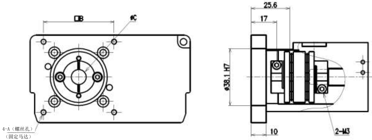
【ECS-10-※※※※※-E】（马达大小：B <□56>）
