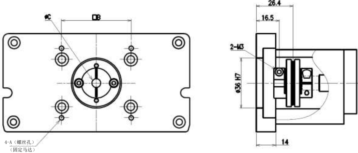
【ECS-14-※※※※※-E】（马达大小：C <□60>）
