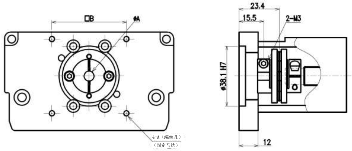
【ECS-12-※※※※※-E】 （马达大小：B <□56>）
