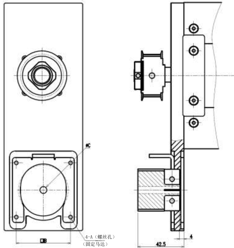
【ECS-14※※※※※- R/L/D】（马达大小：C <□60>）
