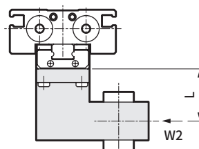
横向弯曲力矩 M2(N \cdot m) = W2 \times L
