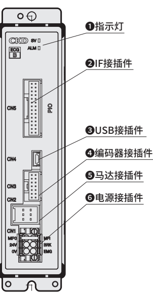
【面板说明】
