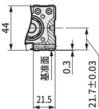
C-C截面 (详图)
