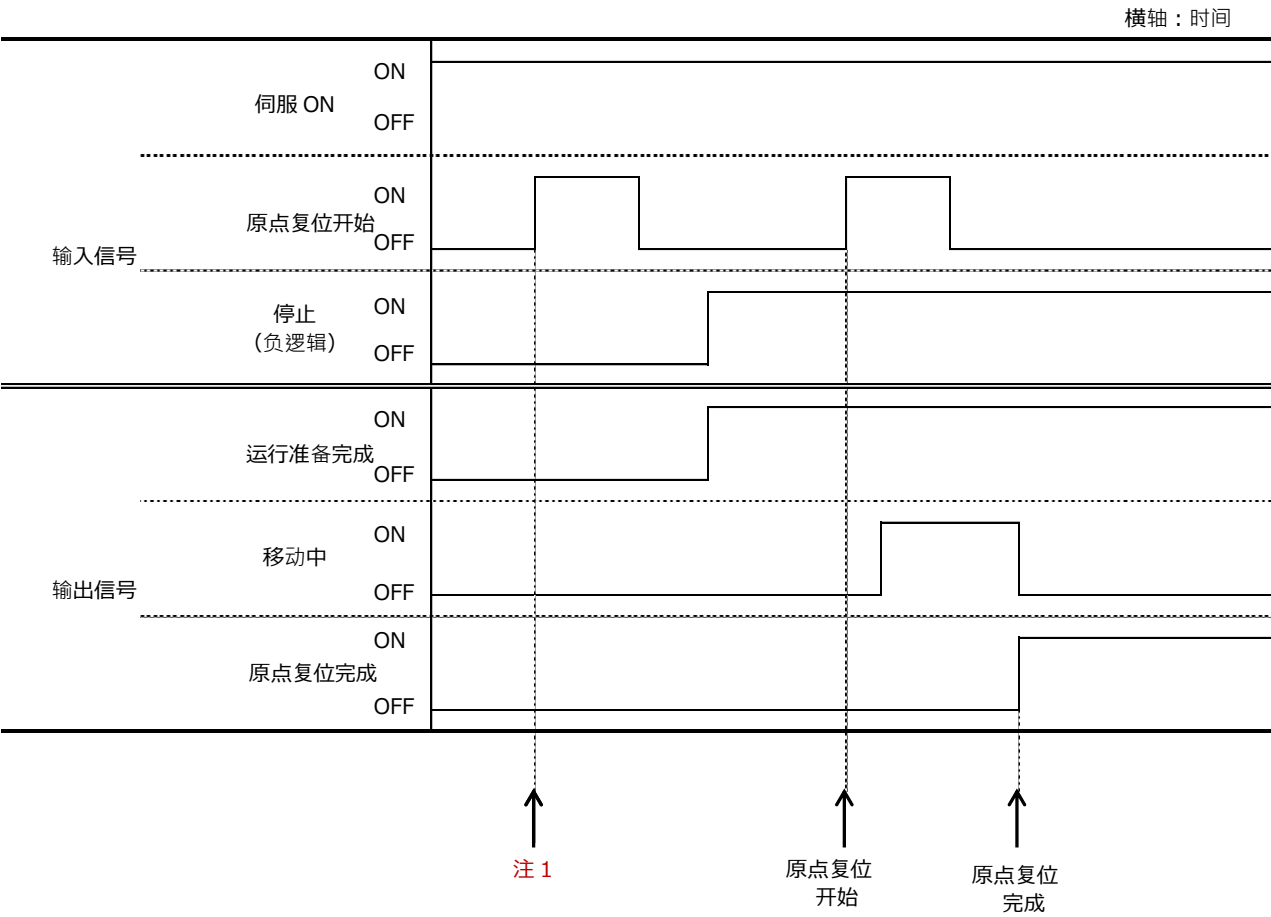
<时序图>
