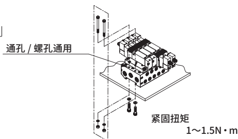
安装方法
