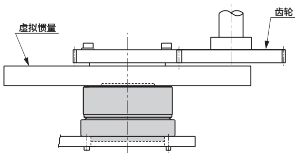
[图5] 虚拟惯量安装示例3
