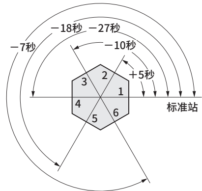
分度精度测定示例
