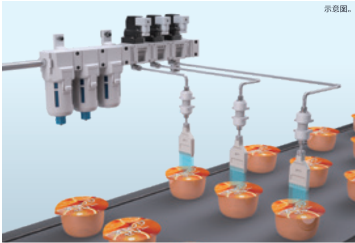
扁平型空气喷嘴
