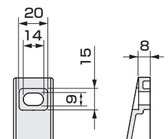
支撑件放大图
