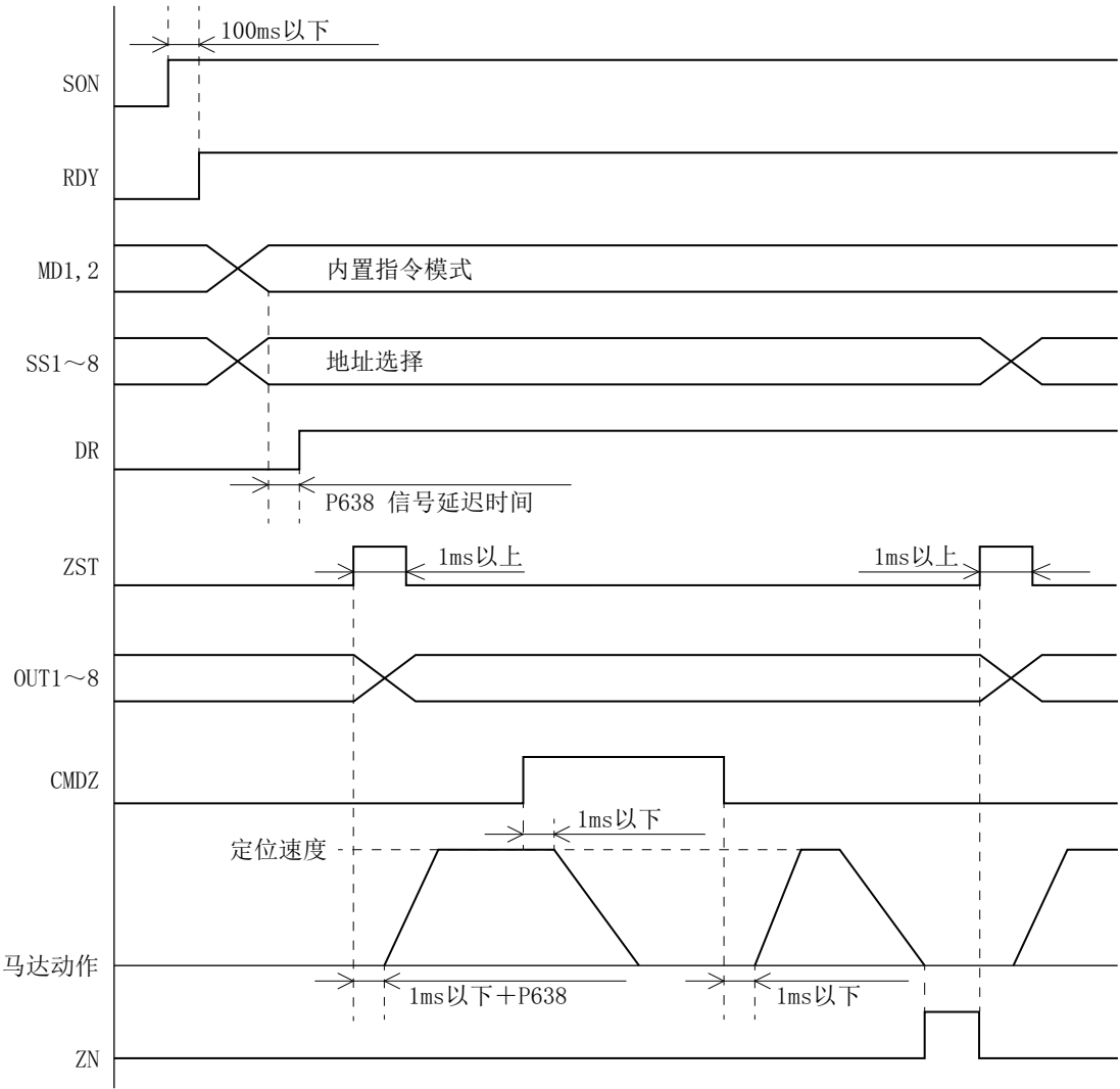
图5-21 INDX命令时序图
