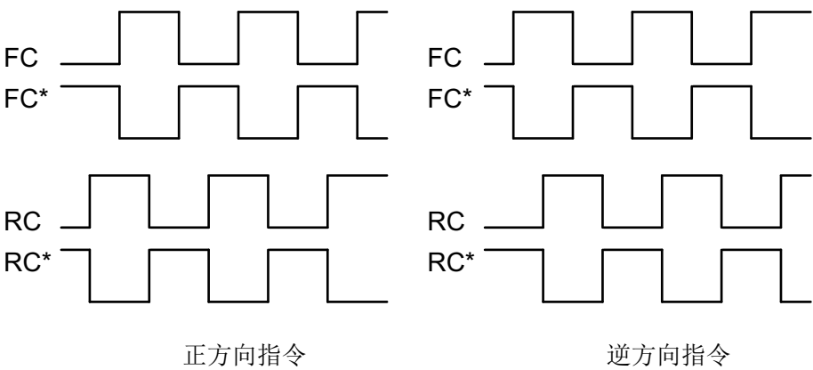
图3-3 90° 相位差信号
