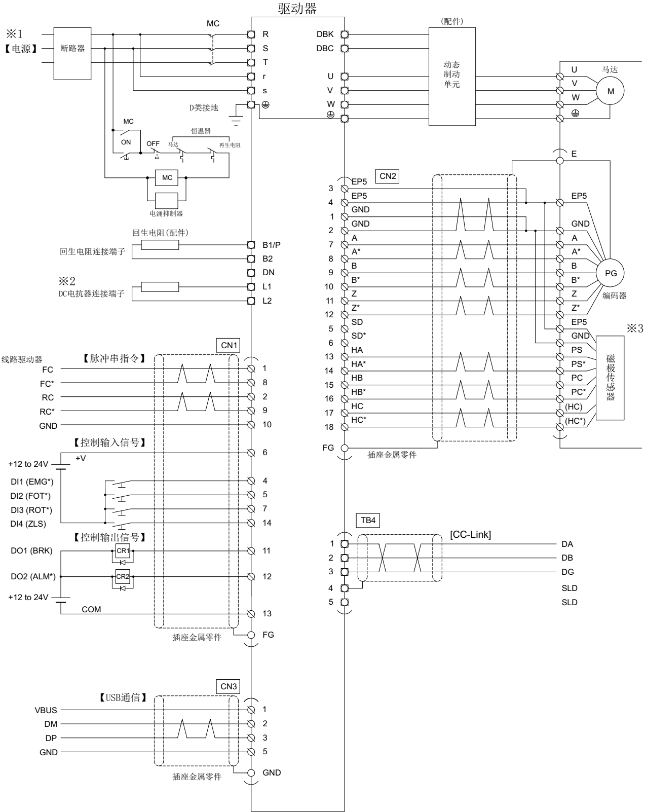
图3-1 外部连接图
