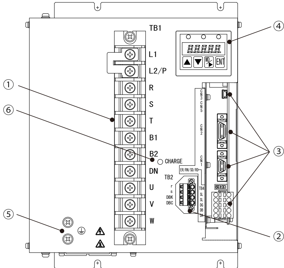
图13-10 7kW驱动器主体正面图（Type5）
