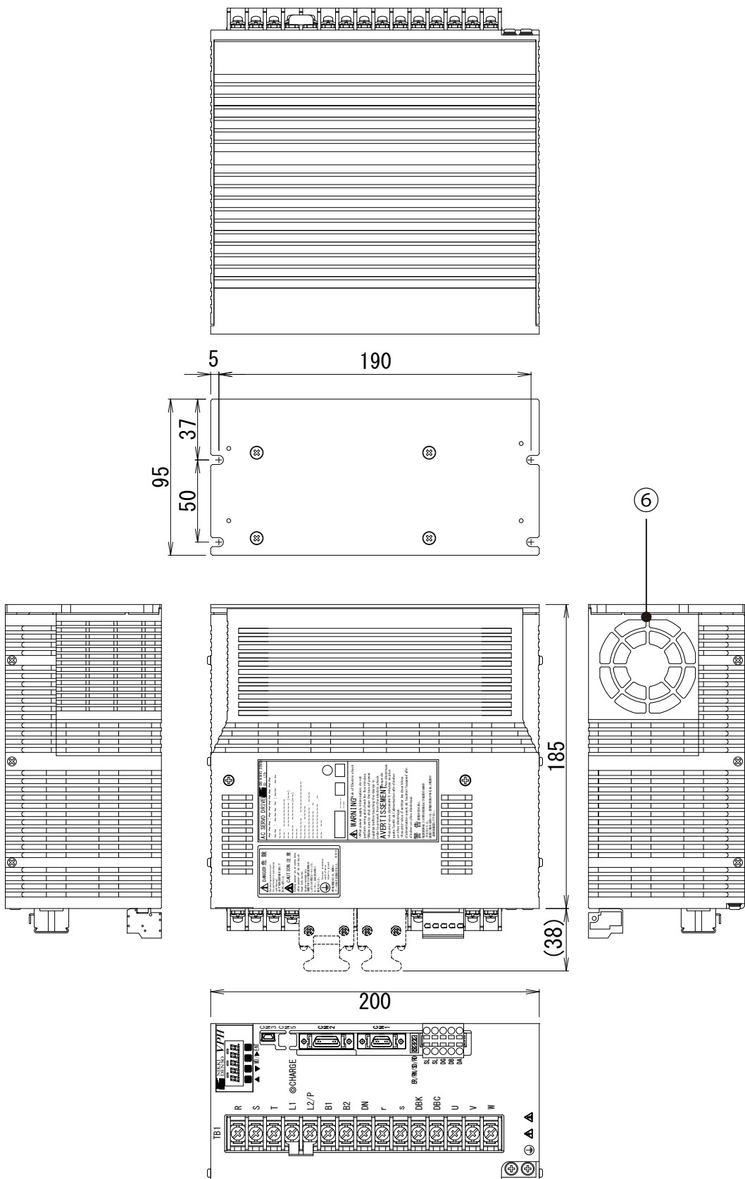
图13-5 1.5kW、2.2kW驱动器主体外形图（Type3）
