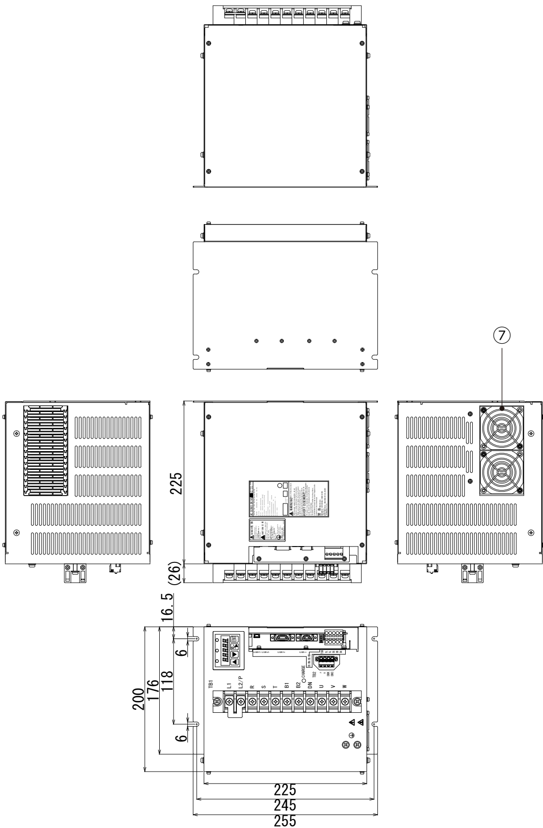
图13-9 7kW驱动器主体外形图（Type5）
