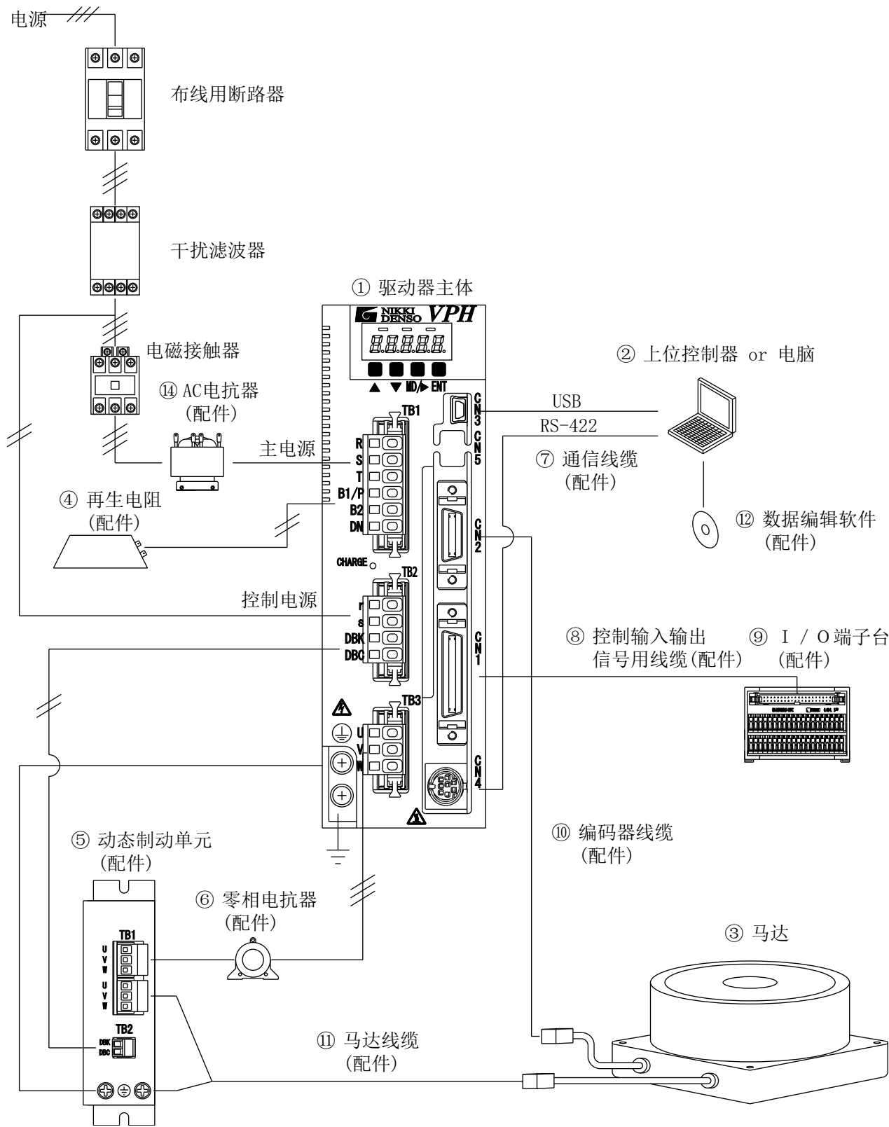
图1-1 800W级以下VPH HA类型 系统构成
