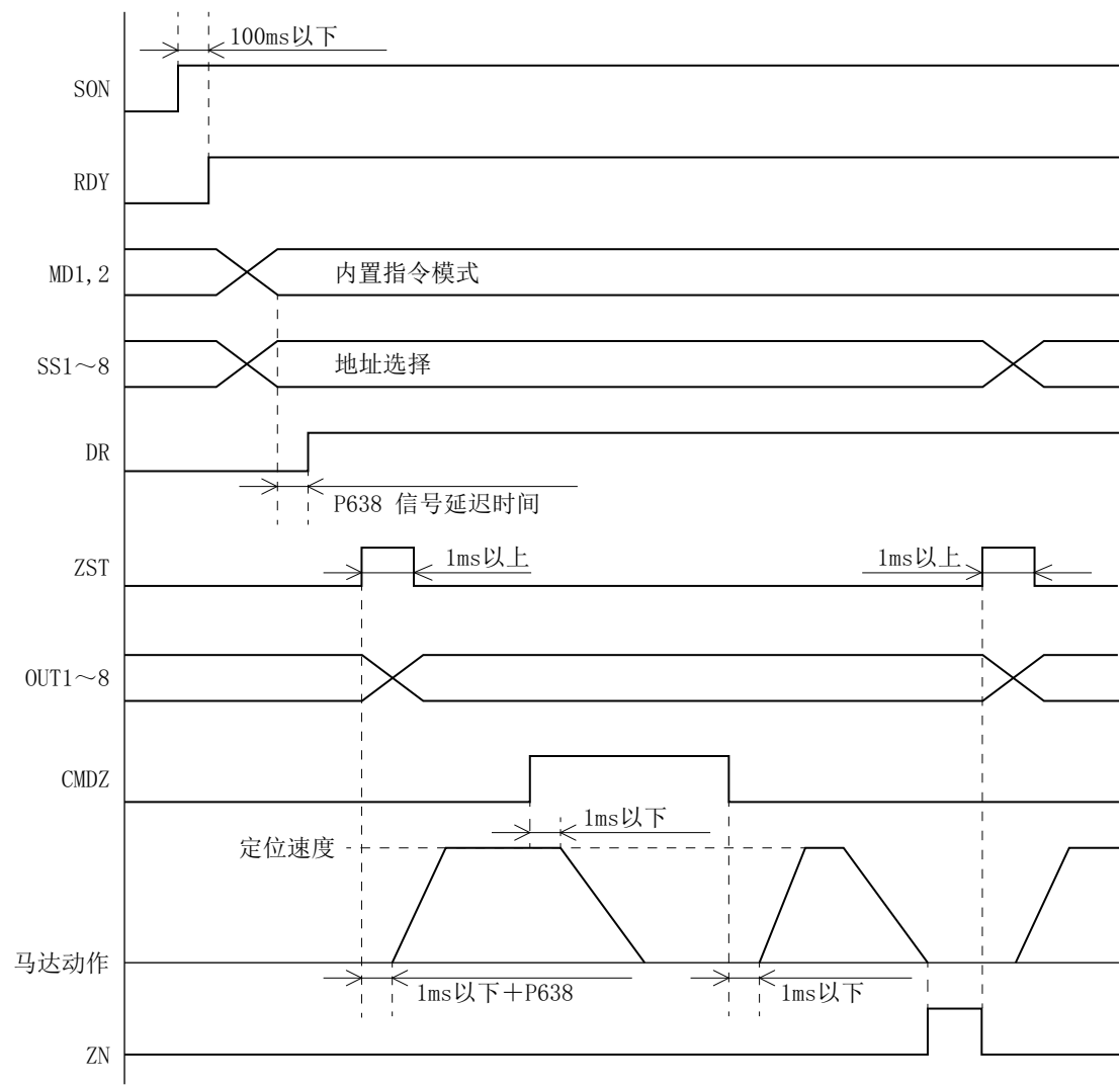
图5-30 INDX命令时序图
