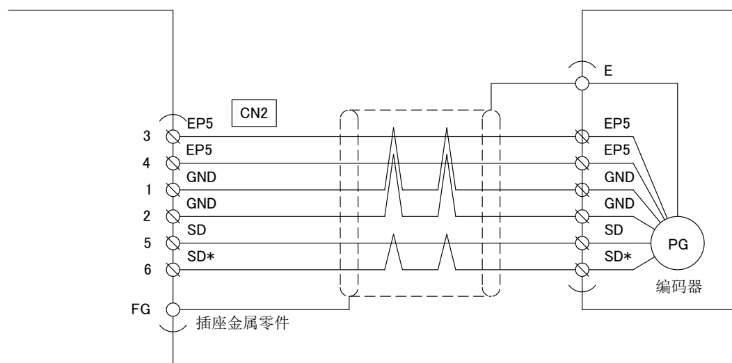
图3-2 串行编码器连接图
