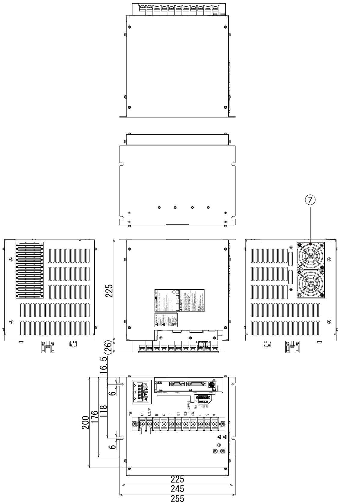
图13-9 7kW驱动器主体外形图（Type5）
