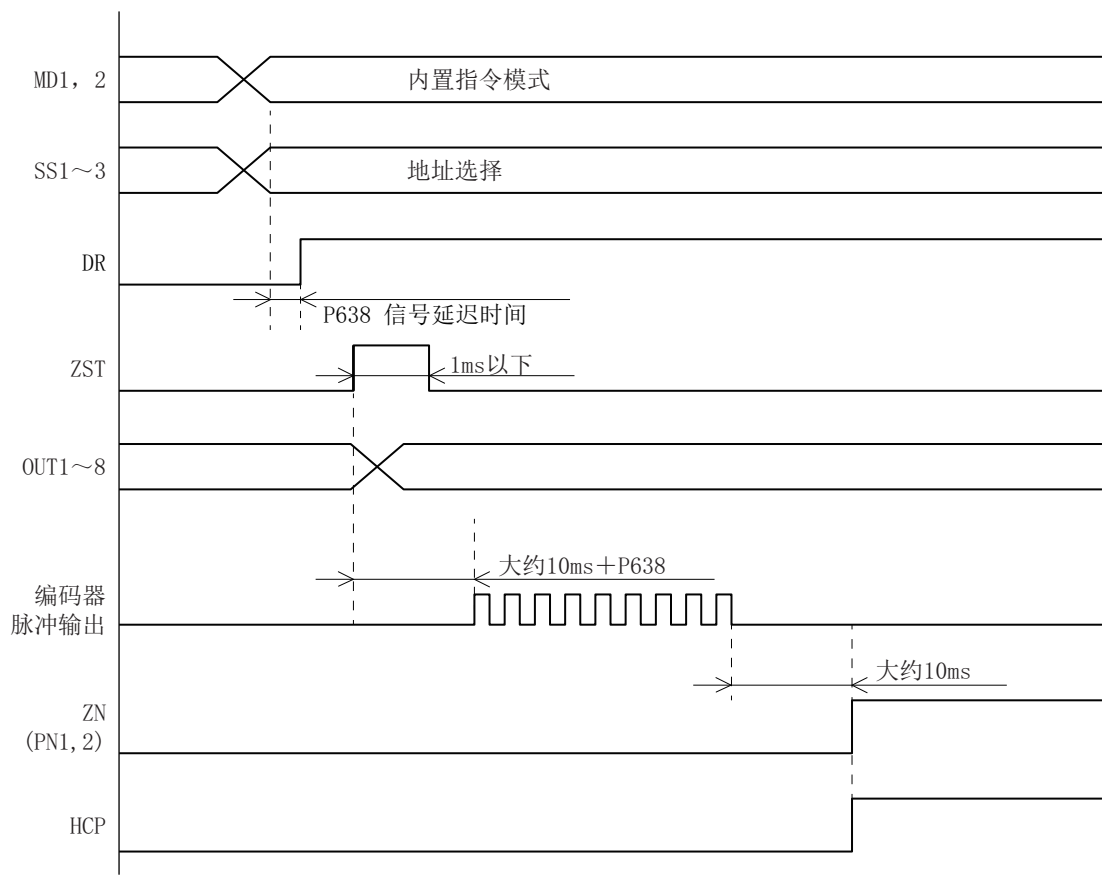
图 5-29 OUT POS 时序图
