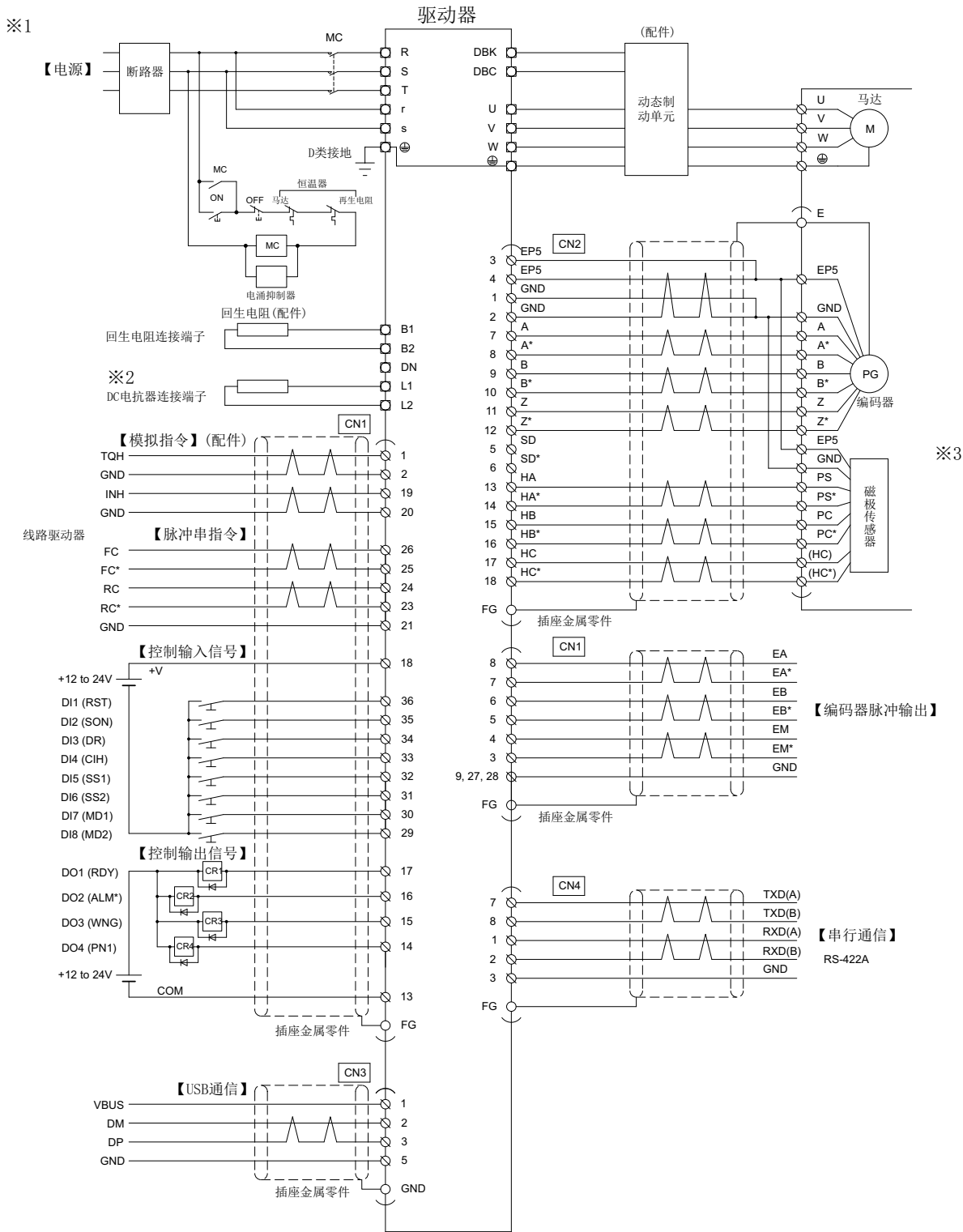
图3-1 外部连接图
