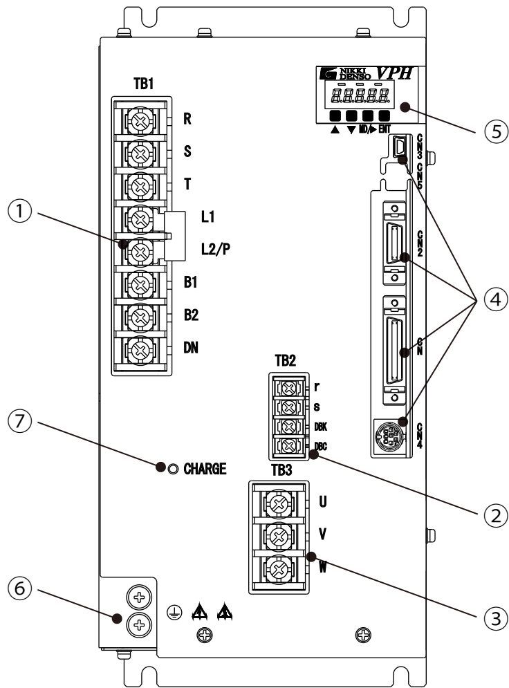
图13-8 3.3kW驱动器主体正面图（Type4）
