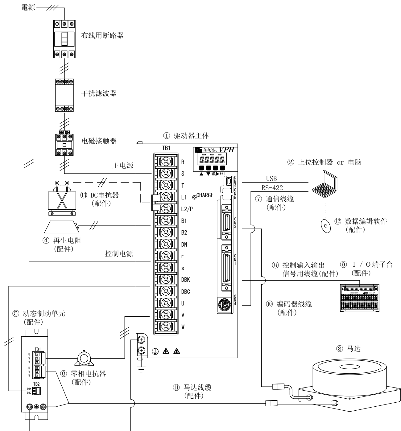
图1-2 1.5kW级以上VPH HA类型 系统构成
