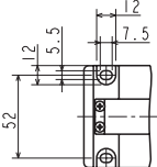
X轴长孔部详图
