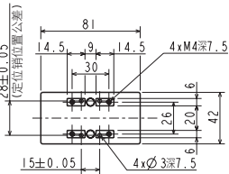
Y轴滑块部详图
