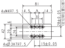
Y轴滑块部详图
