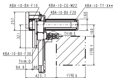
KBA-10-FD-L-●截面 KBA-10-FD-S-●截面
