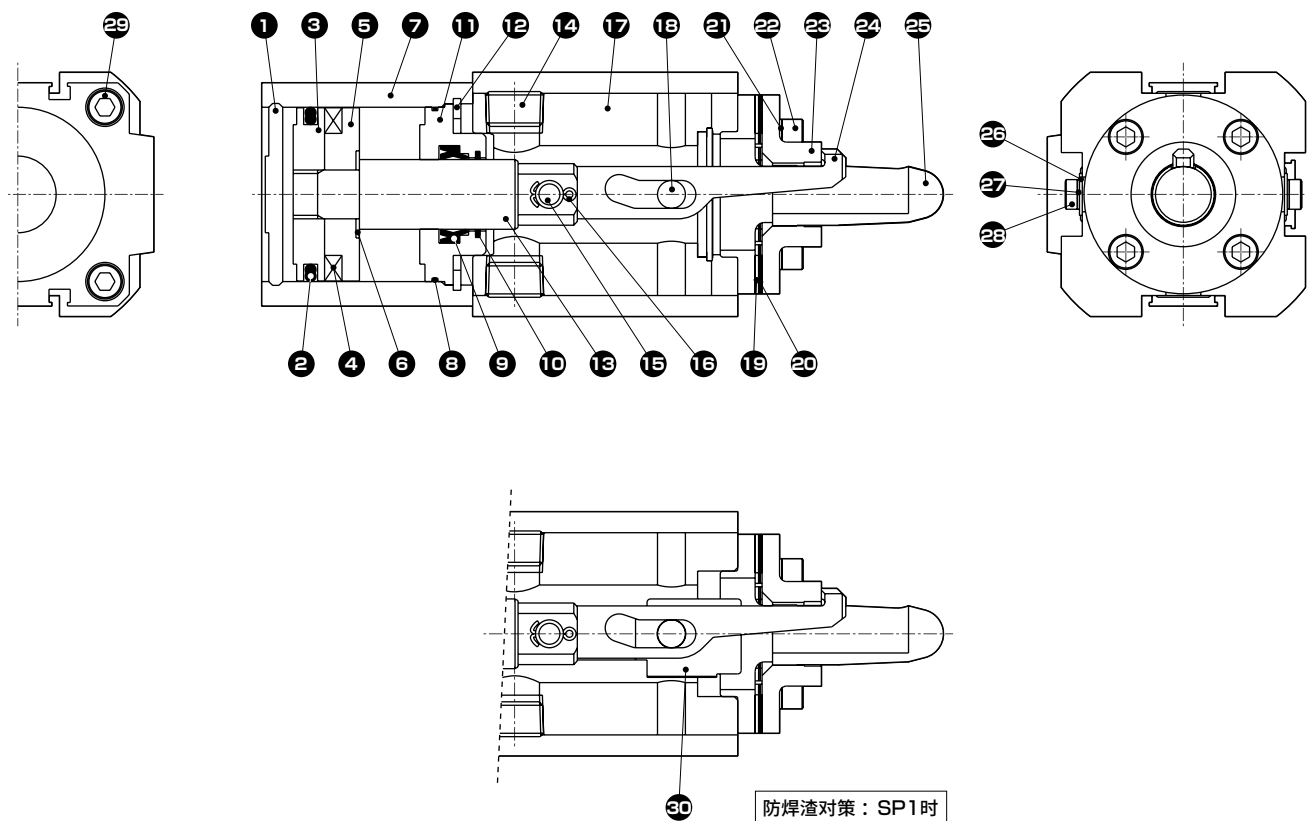
内部结构及部件一览表(PCC-C1、PCC-C2)
