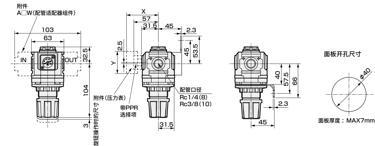
外形尺寸图
