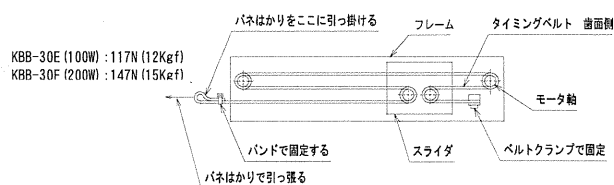
モータ下向き (BU) タイプの場合 (フレームカバー上面よりみた図です)
