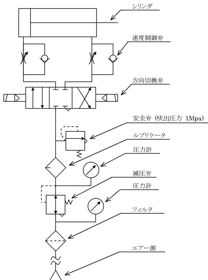
< 基本空気圧回路図 >
