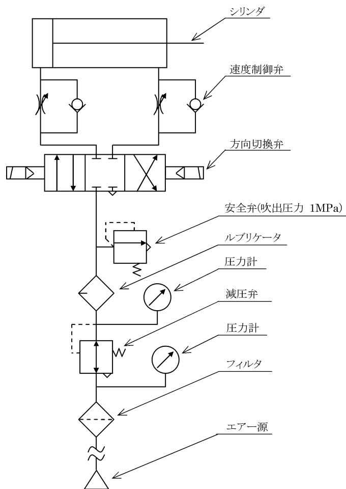
&lt; 基本空気圧回路図 &gt;
