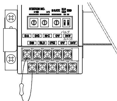
例) DA・DB 間に抵抗を接続した場合
