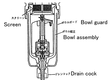
ドレントラップ内部構造 Inside structure of drain trap
