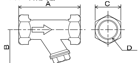
ストレーナ外形寸法
