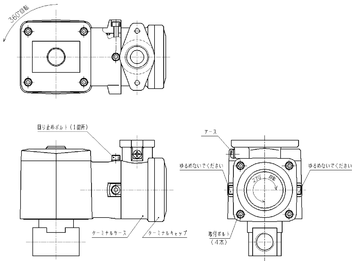
(図6) 端子箱の配線取り出し方向
