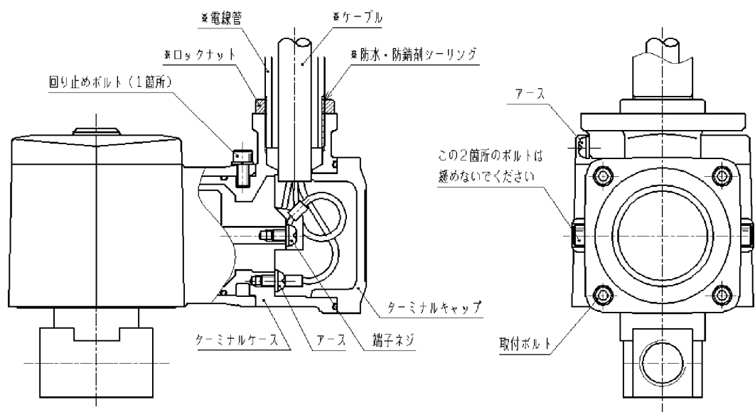
(図4) 電線管ねじ結合式の結線方法の事例
