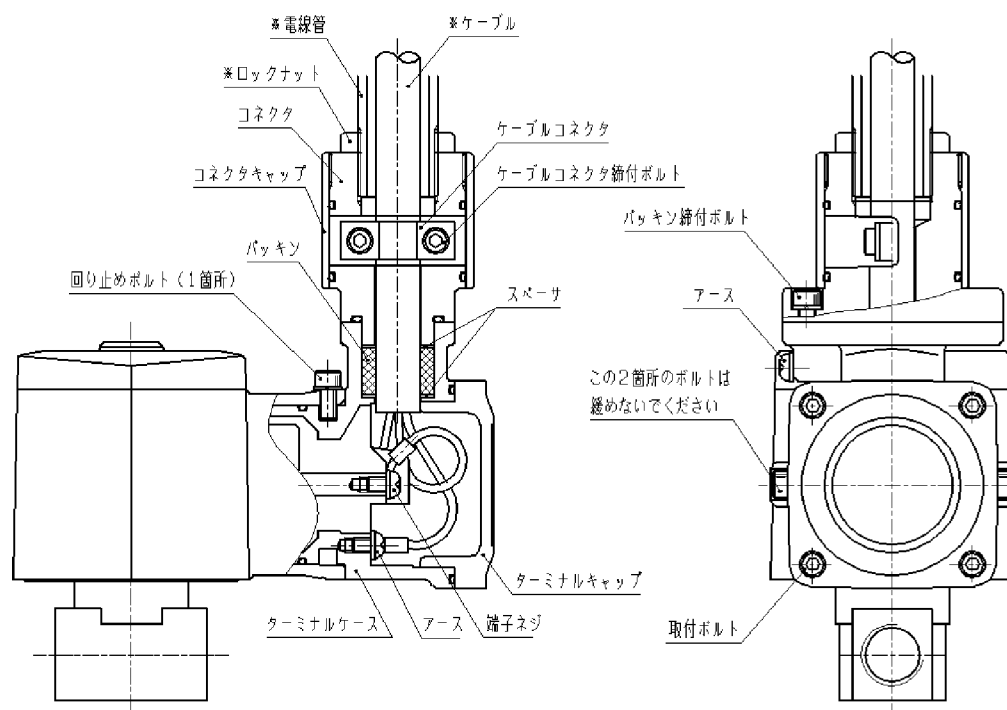
(図5)耐圧パッキン結合式の結線方法の事例
