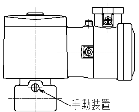
(図7) 手動装置の操作方法
