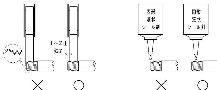
(図3)シール剤の塗布方法
