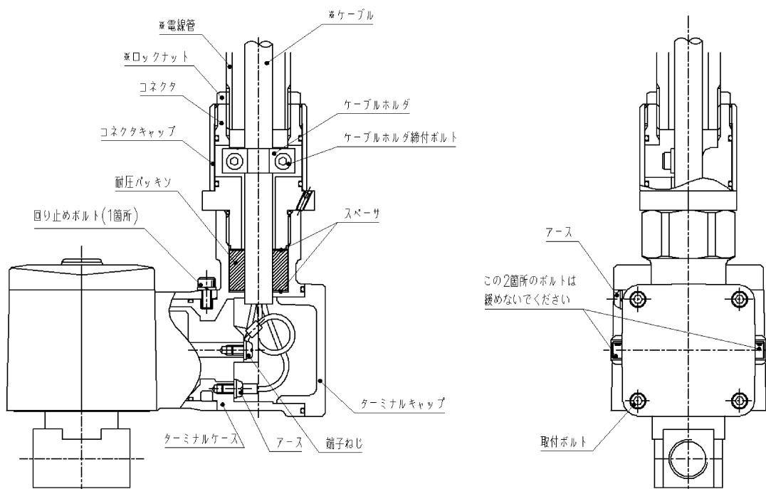
(図4) 耐圧パッキン結合の結線方法の事例
