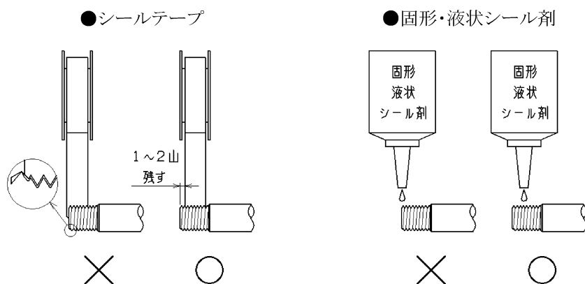
(図3) シール剤の塗布方法
