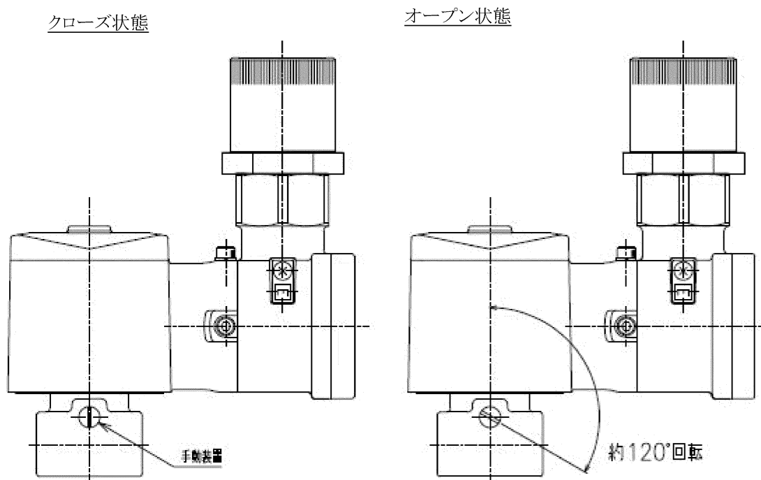
(図6) 手動装置の操作方法
