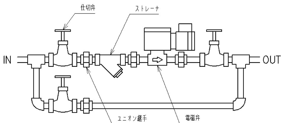
(図1) バイパス回路
