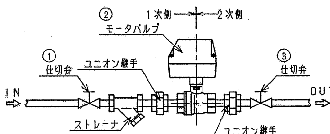
（図 8 配管図）
