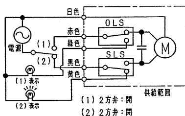
( 図 14 閉作動終了時 )
