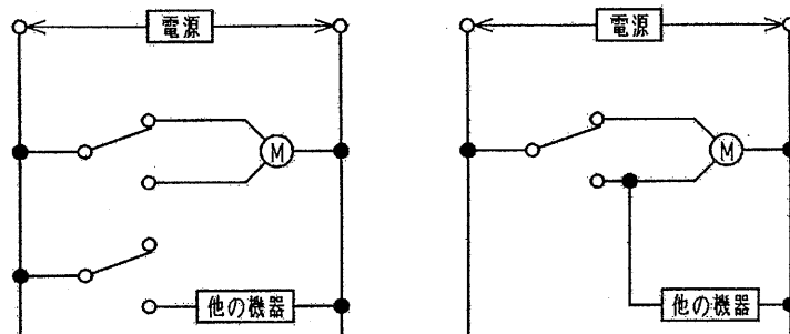
(図6 他の機器との結線方法)
