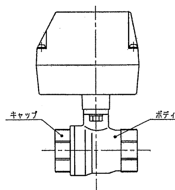
(図3 外観図)
