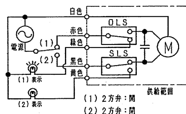
( 図 15 開作動終了時 )
