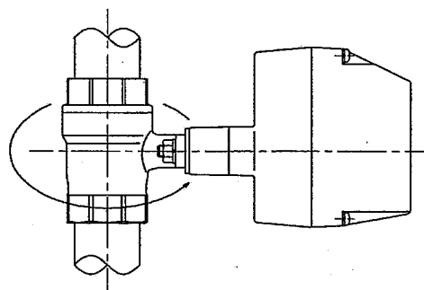
<垂直配管の場合>
