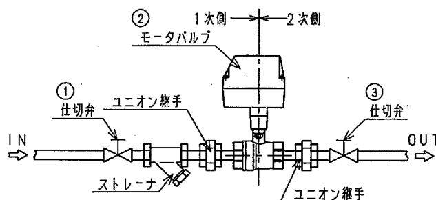
（図 6 配管図）
