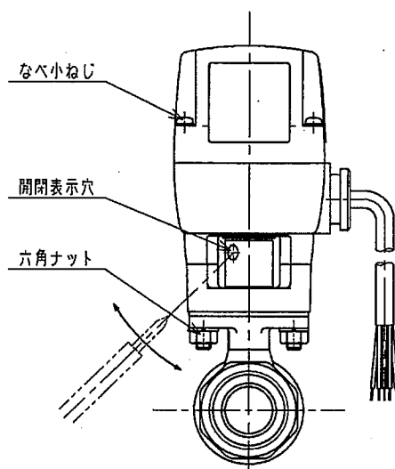
( 図 8 外観図 )
