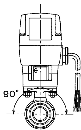
<水平配管の場合>
