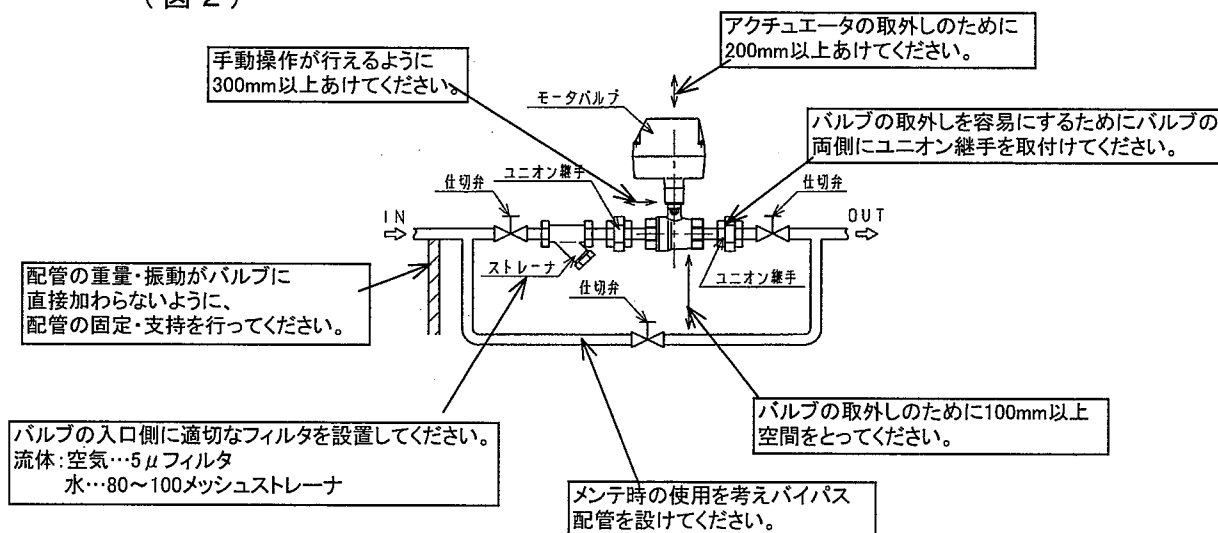
（図2 配管モデル）
