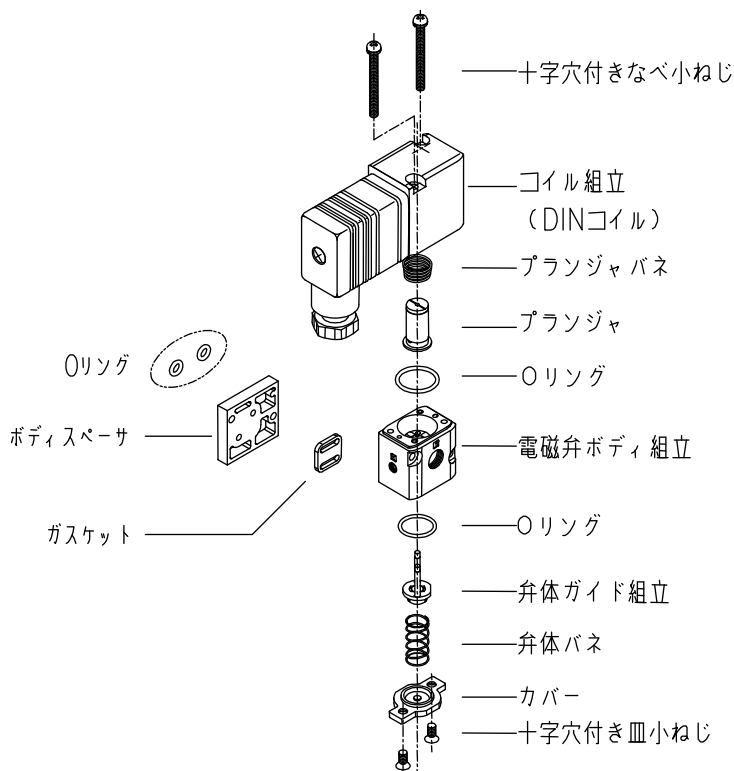
(図5-1)パイロット用電磁弁の分解図
