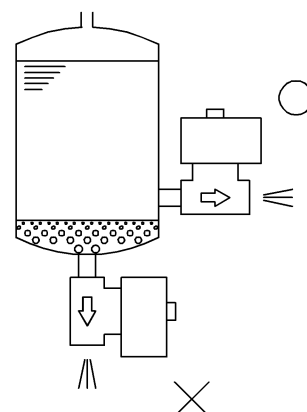
(図1) タンクからの排出回路
