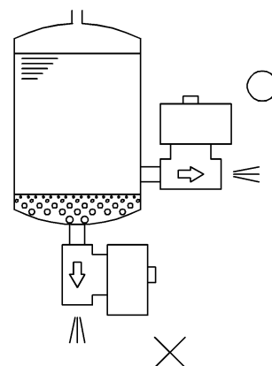
(図1) タンクからの排水回路
