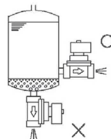
(図2) タンクからの排水回路
