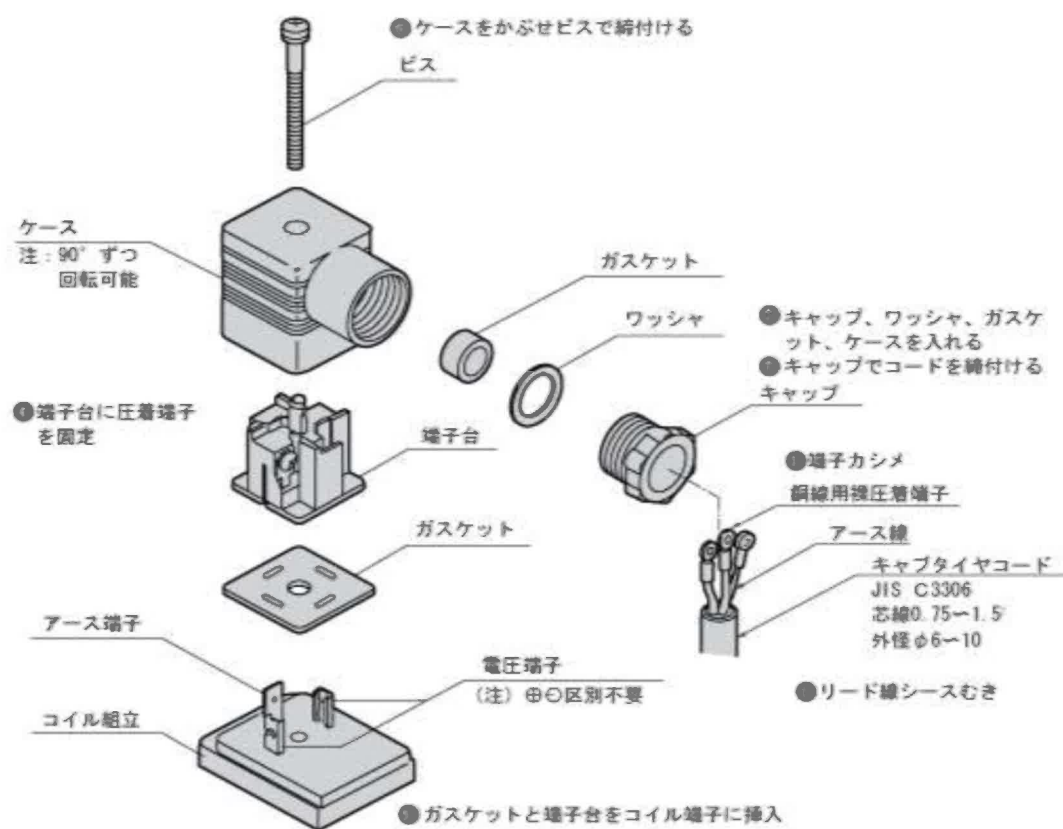
(図5) DIN端子箱の結線方法
