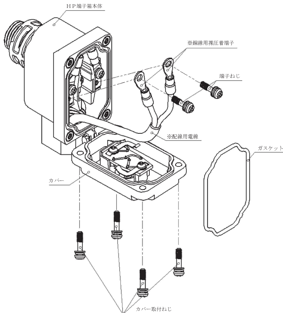
(図6) HP端子箱の結線方法
