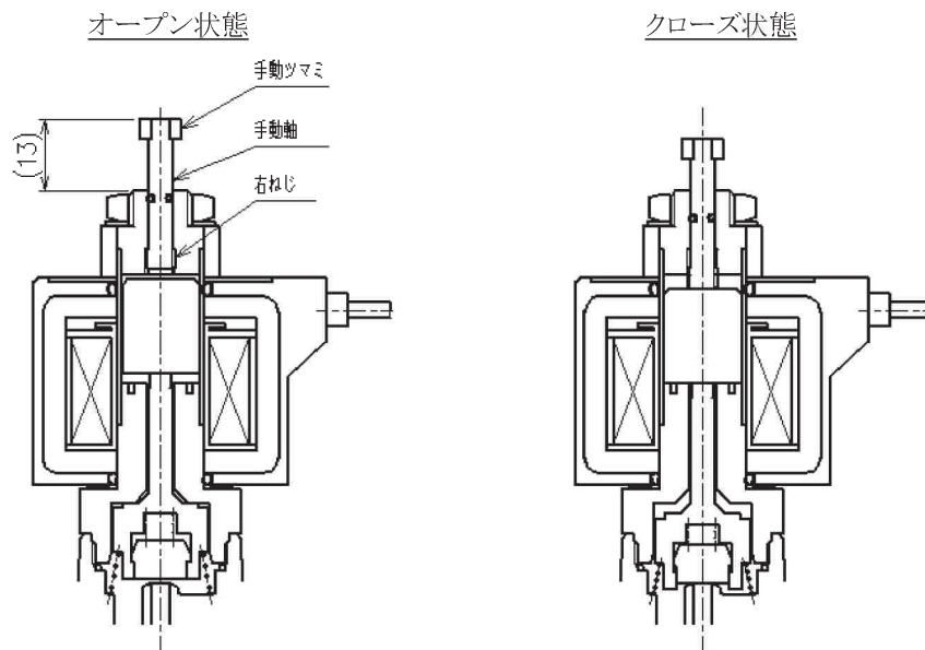
(図8) 手動装置の操作方法
