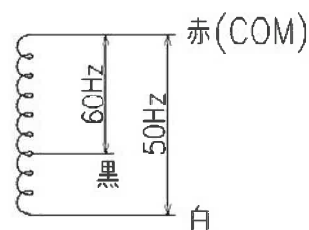
(図5) 3本リード線の結線方法
