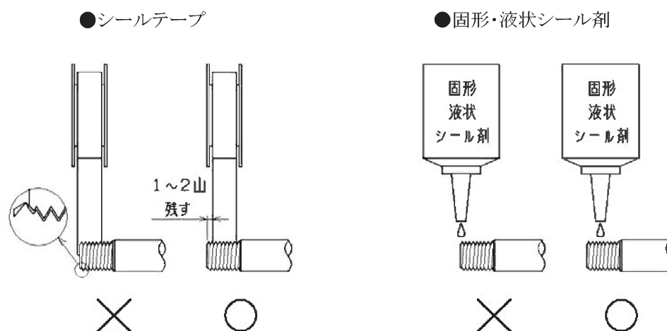
(図4)シール剤の塗布方法
