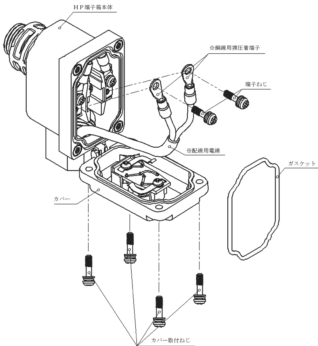
(図6) HP端子箱の結線方法
