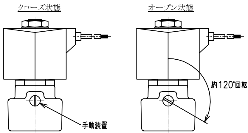
(図4) 手動装置の操作方法
