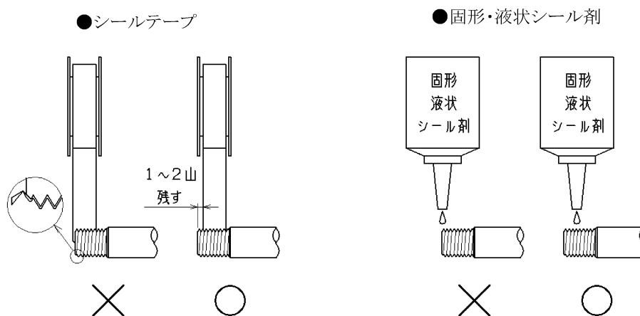
(図1)シール剤の塗布方法
